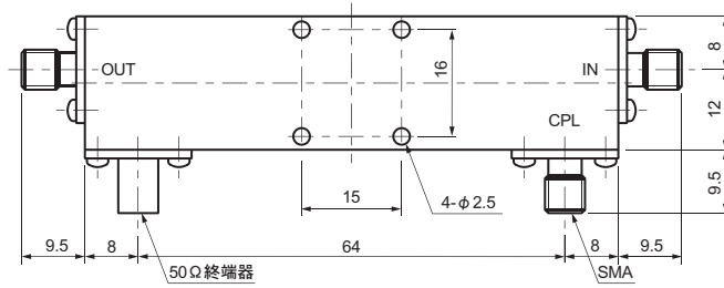
Fig. 1 SMA Type
