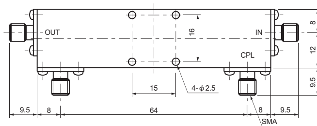
Fig. 2 SMA Type
