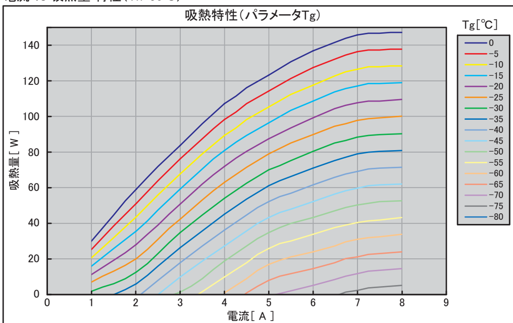
電流 vs 吸熱量 特性 (Th=50℃)
